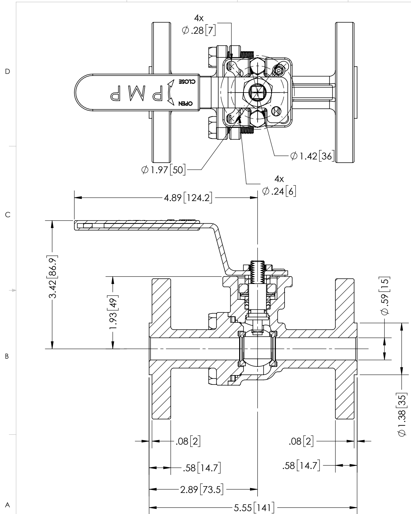
SECTION A-A
